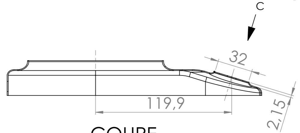
COUPE B-B
